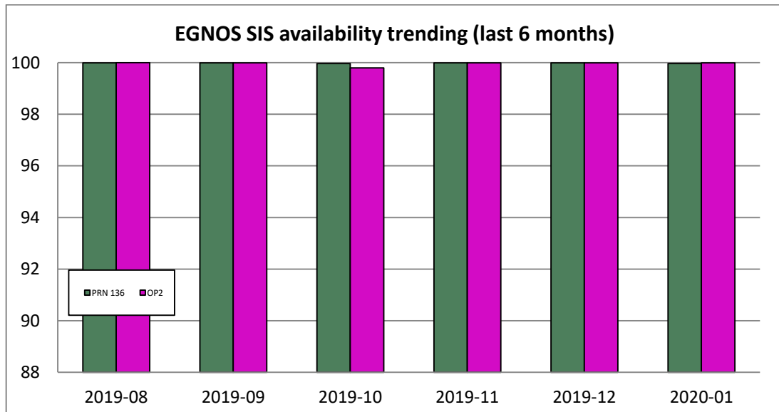
Figure 2 – Trend of EGNOS SIS Availability per GEO.
